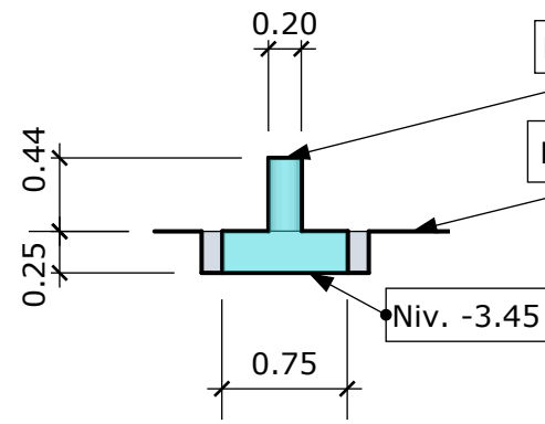
Coupe non hors gel 1:50
