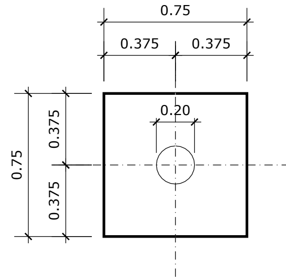
Vue en plan socle 1:20
